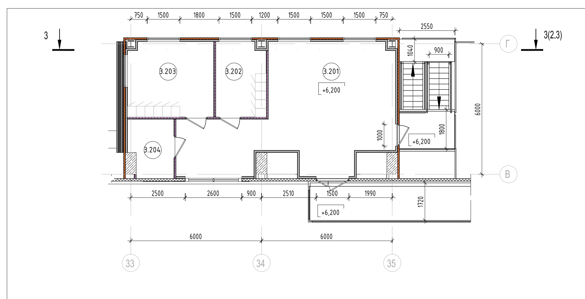
План на отм. +6,230 в осях 36-39/В-Г
