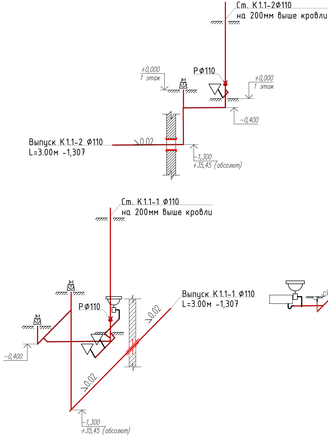
Схема водоотведения выпуск K1.1
