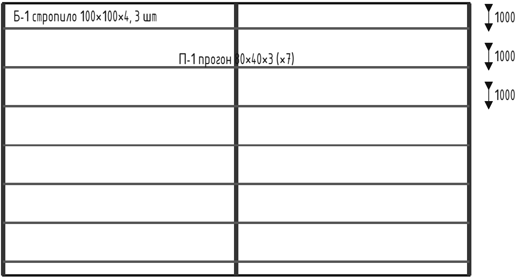
Схема кровельной обрешётки. Прогоны 80×40×3, шаг 1000
