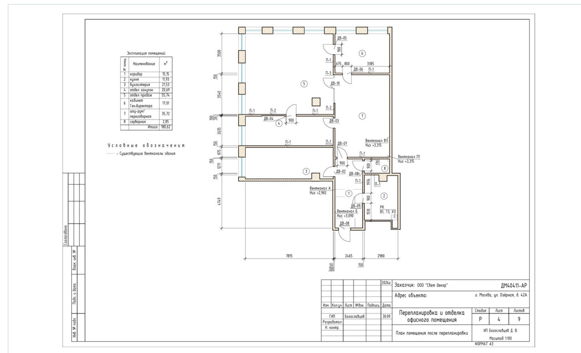
План после перепланировки • стр. 4
