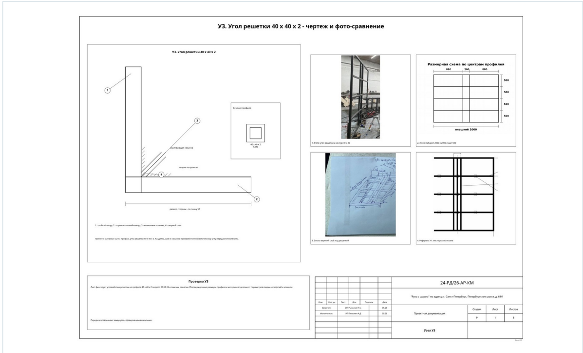
Узел УЗ: чертёж и фото • стр. 1
